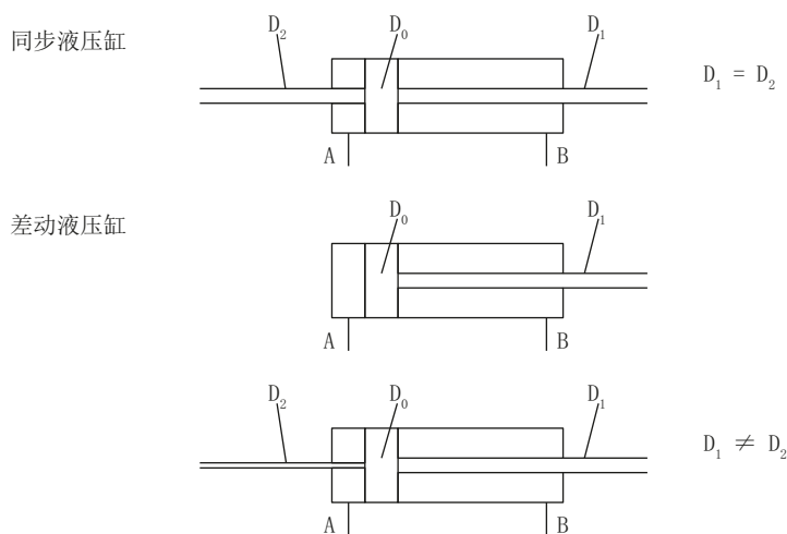
图 A-19 液压缸原理图
