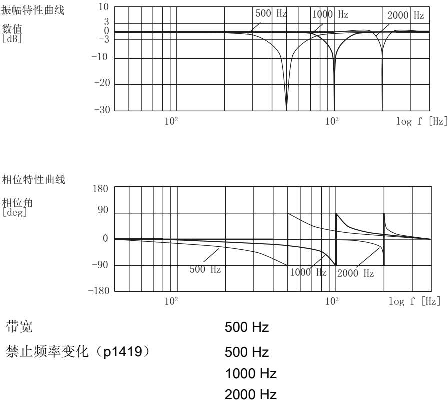
图 5-4 未衰减带阻的频率响应
