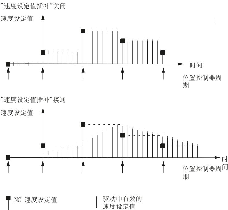
图 5-2 速度设定值插补
