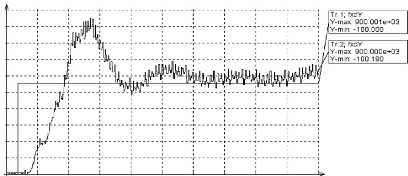
图 4-49 速度控制环设定值阶跃时间特性（示例）
