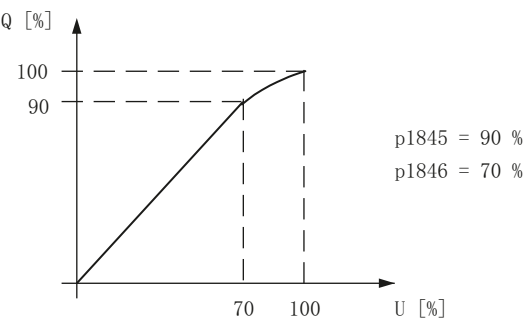
图 5-17 拐点补偿示例
