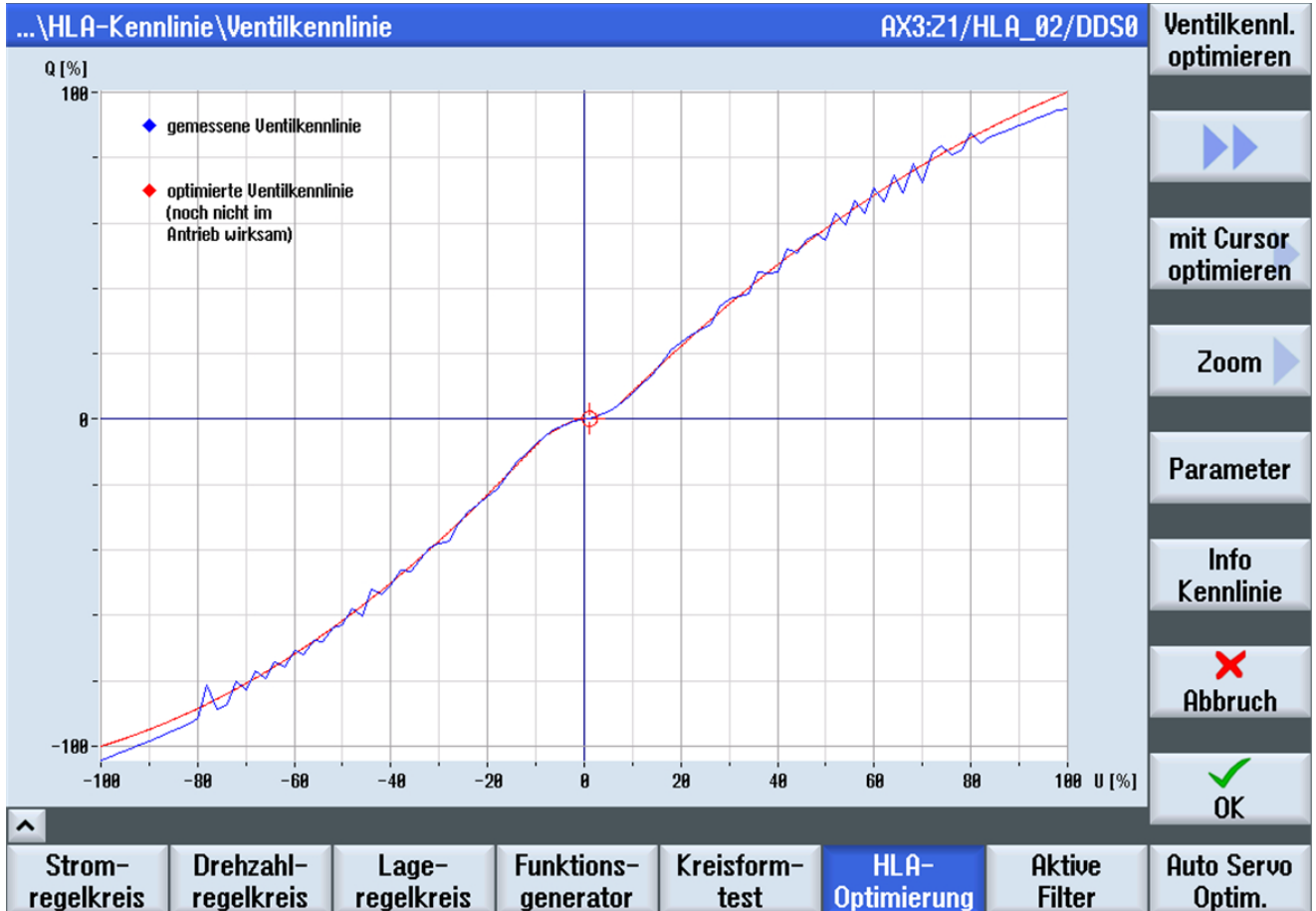
图 4-32 阀门特性曲线图形优化
