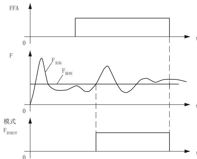
图 5-11 通过关闭“运行到固定挡块”功能撤销力控制
