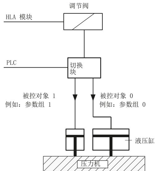
图 5-1 参数组切换示例
