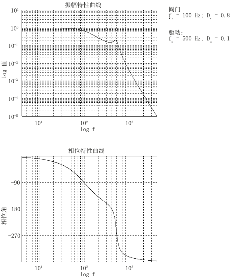
图 4-43 被控对象的频率响应特性 ( f_{\text{阀门}} \ll f_{\text{液压缸}} )
