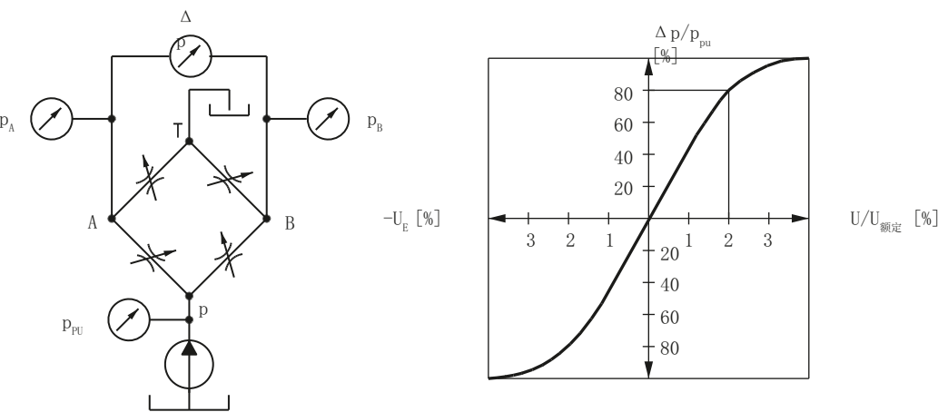
图 A-5 压力放大
