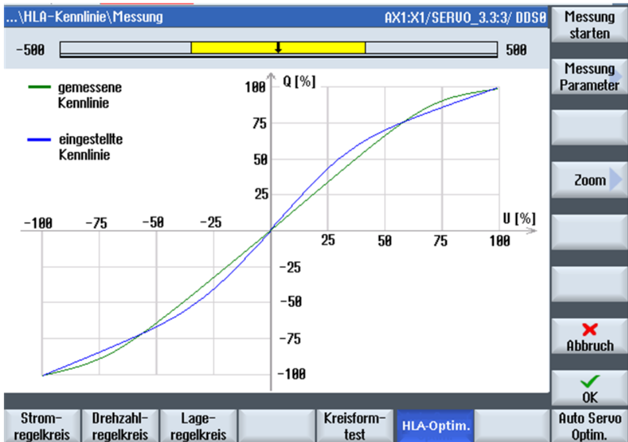
图 4-28 特性曲线：测量
