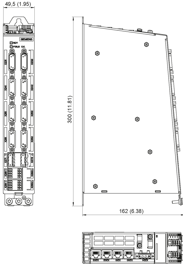
图 6-2 HLA 模块外形尺寸图，所有数据单位：mm 和(inch)
