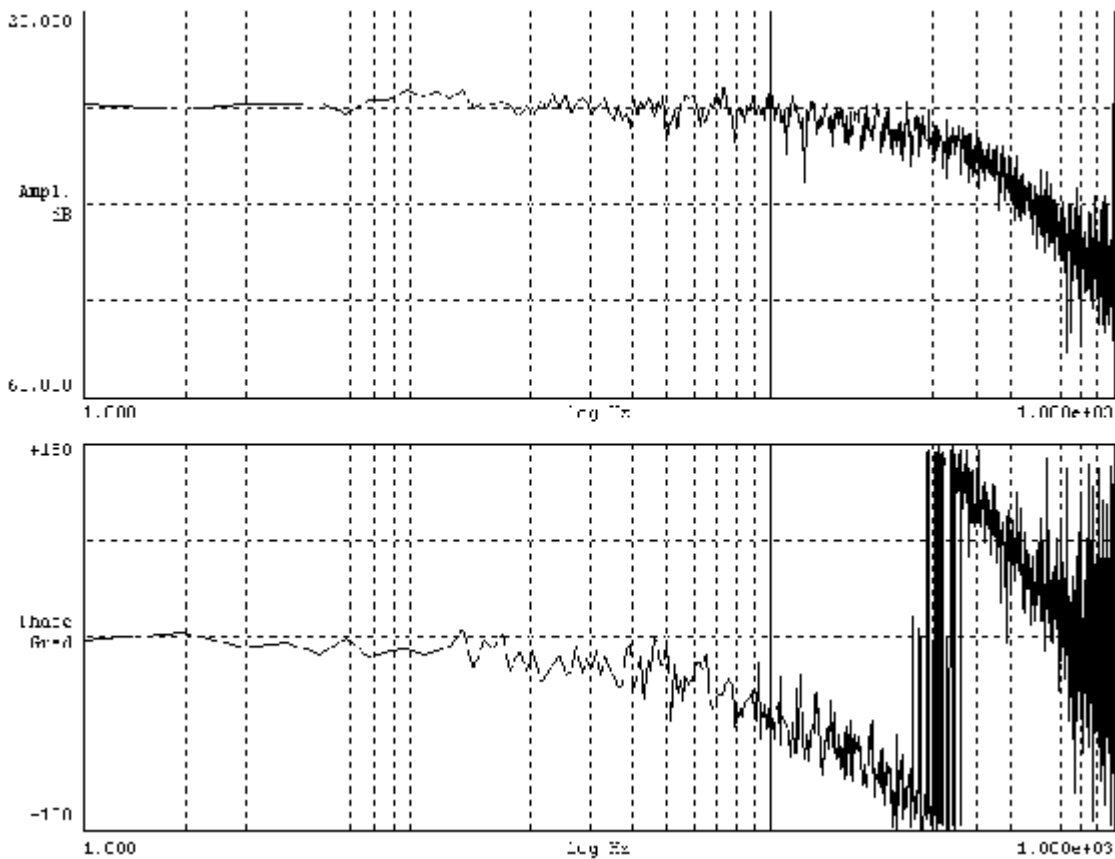
图 4-47 HR 调节阀阀门频率响应 (示例)
