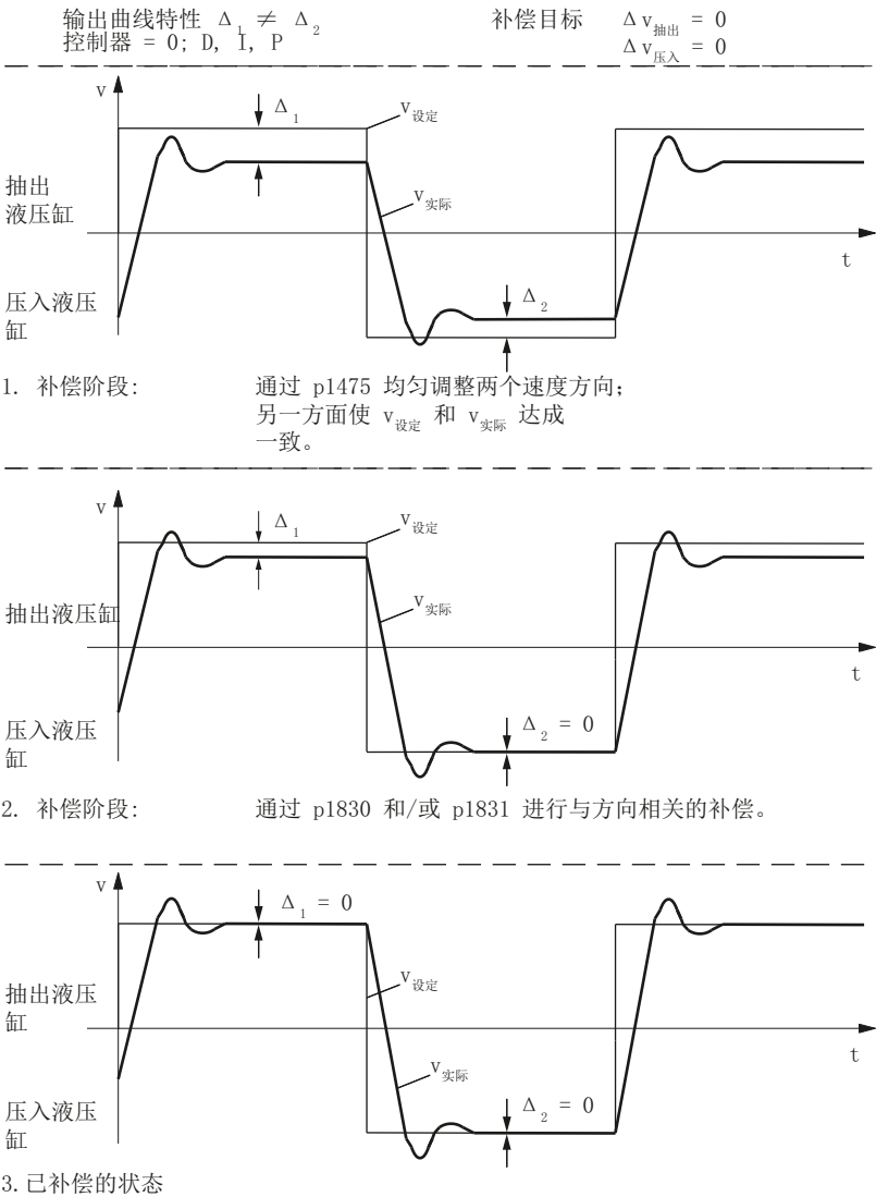
图 4-42 系统增益校准
