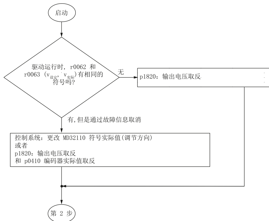
图 4-39 确定调节方向的调试顺序图
