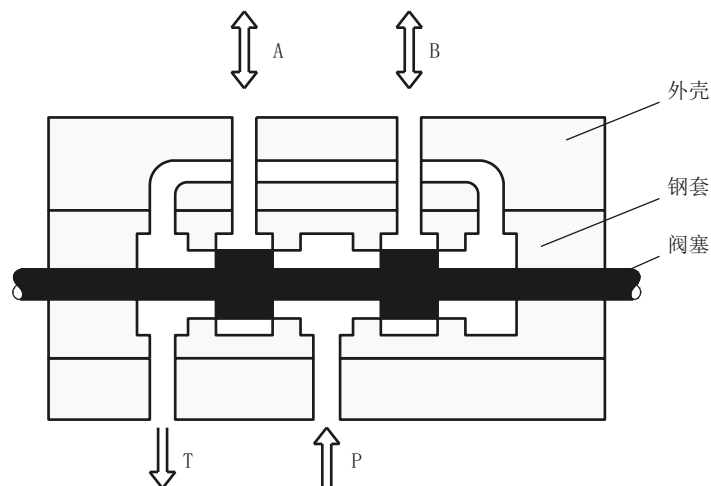
图 A-1 阀塞原理
