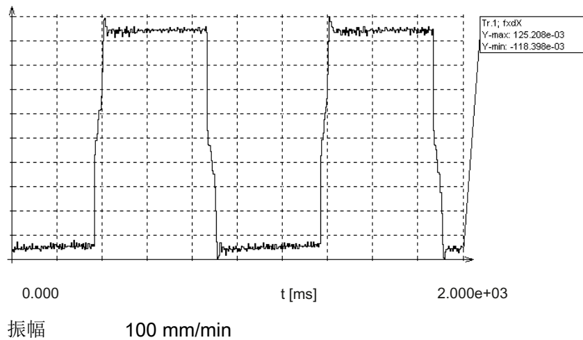
图 4-55 在信号类型为“方波”时，“速度实际值”到速度设定值的跟踪
