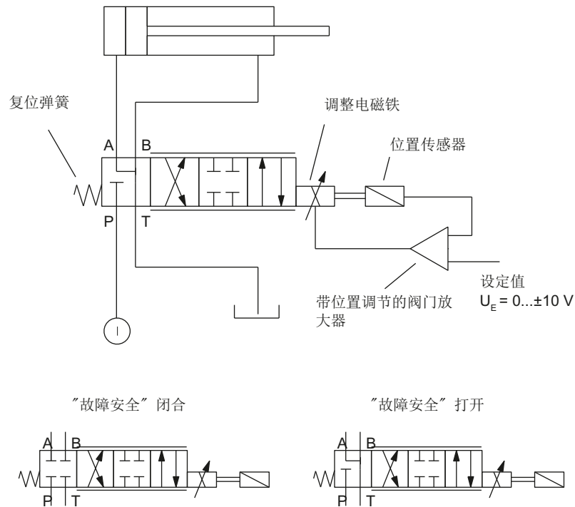
图 A-3 开关符号
