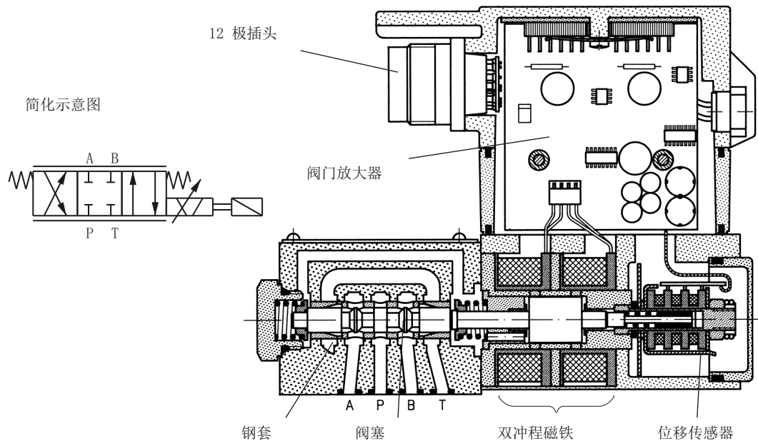
图 A-17 直接控制的 HR 调节阀
