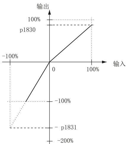
图 4-34 特性曲线表面补偿
