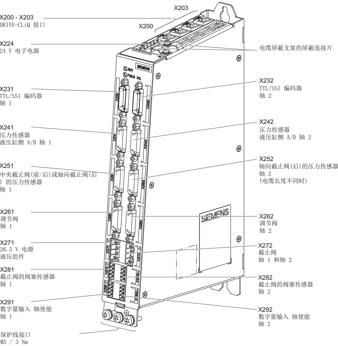
图 6-1 HLA 模块接口一览
