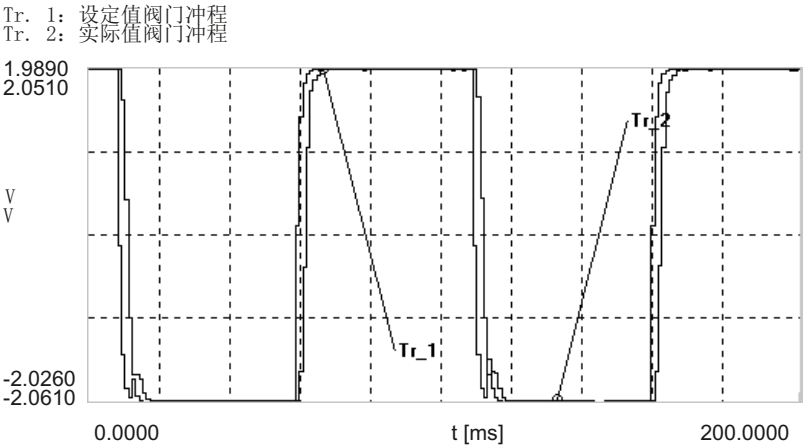
图 4-54 在信号类型为“方波”时，“阀门实际值”到阀门设定值的跟踪
