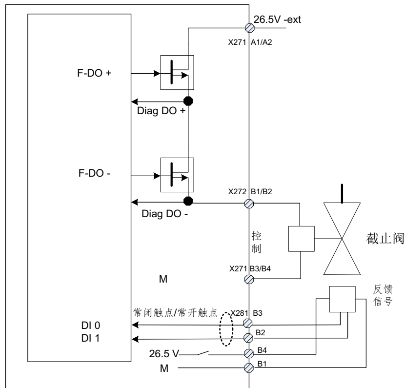
图 3-5 截止阀连接图
