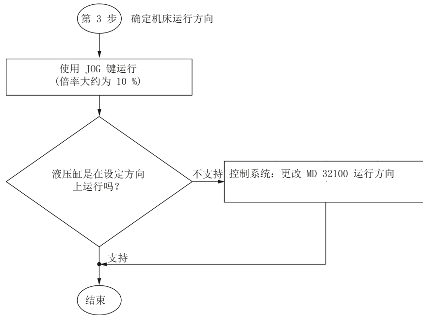
图 4-41 NC 运行方向定义的调试顺序图
