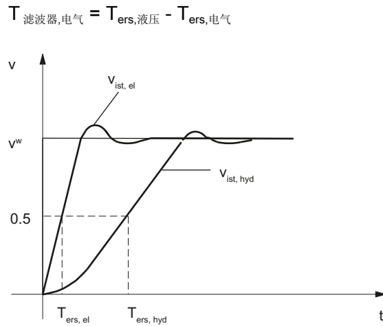
图 4-46 液压/电气插补
