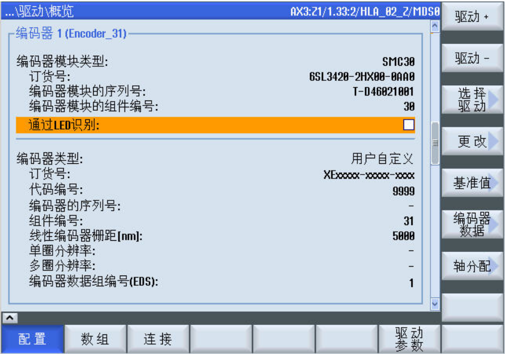
图 4-17 编码器一览
