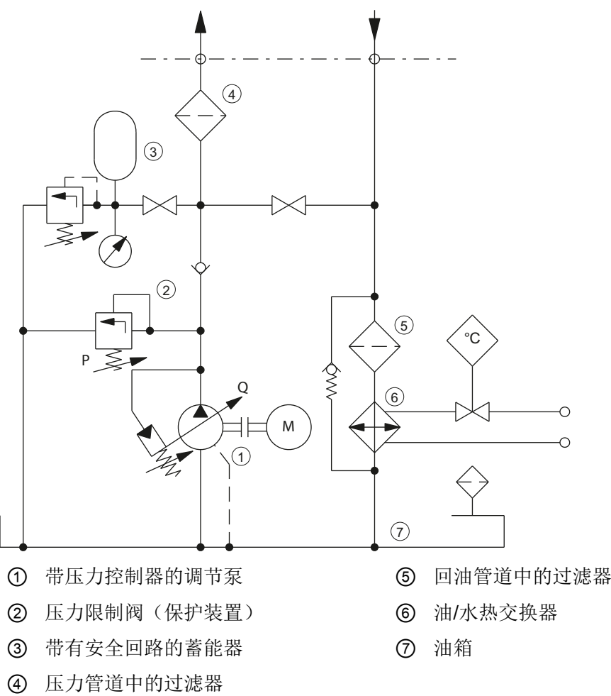
图 3-6 典型液压装置一览
