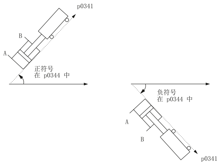
图 5-19 基于 A 侧的驱动安装位置
