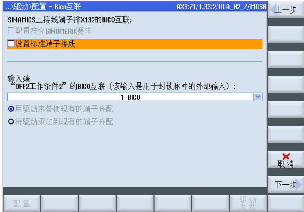
图 4-13 配置 - BICO 互联
