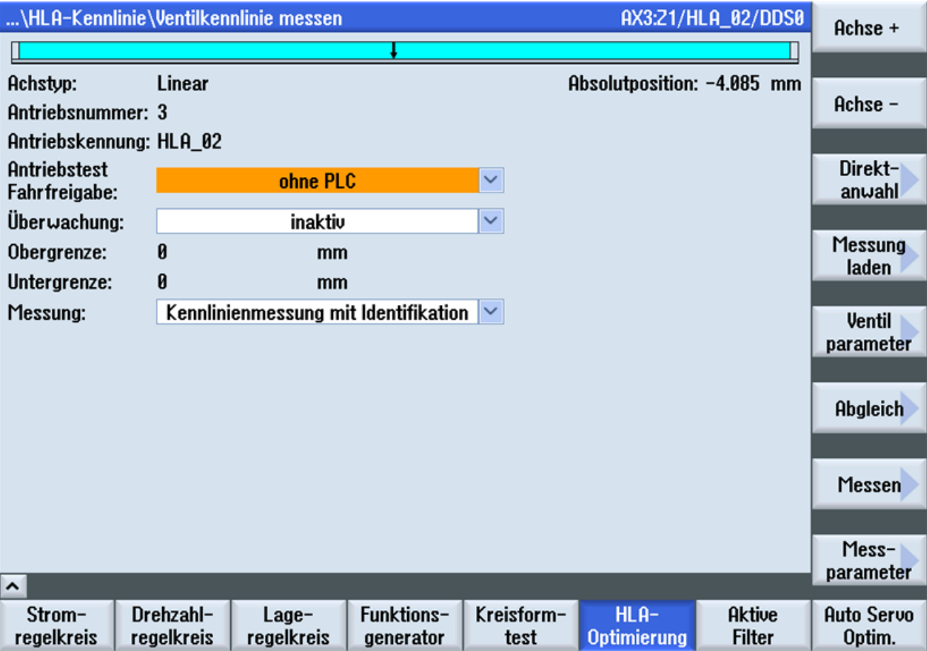
图 4-25 测量阀门特性曲线
