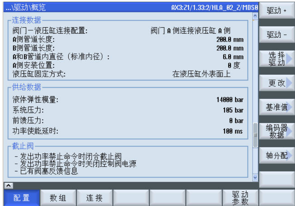
图 4-18 供给单元/截止阀的连接数据一览
