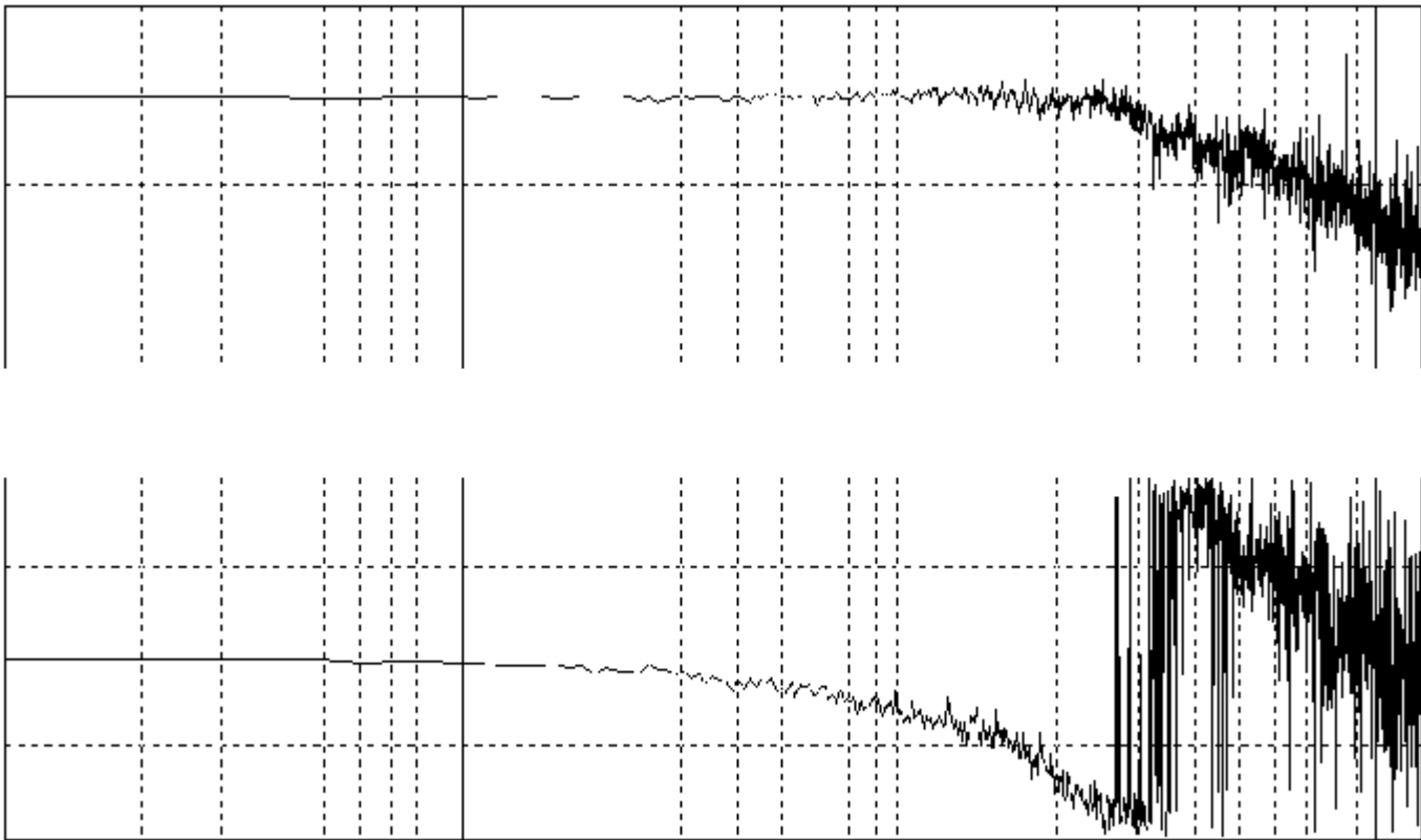
图 4-53 位置控制环测量示例（示例）
