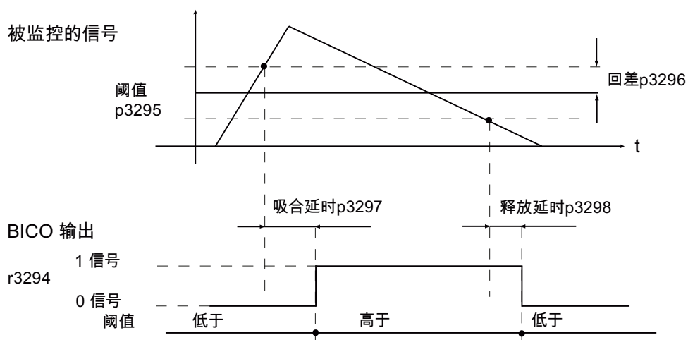
图 5-23 变量报告功能
