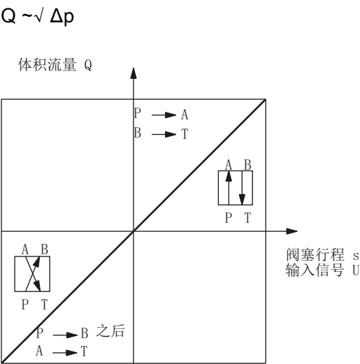
图 A-6 线性体积流量特性曲线
