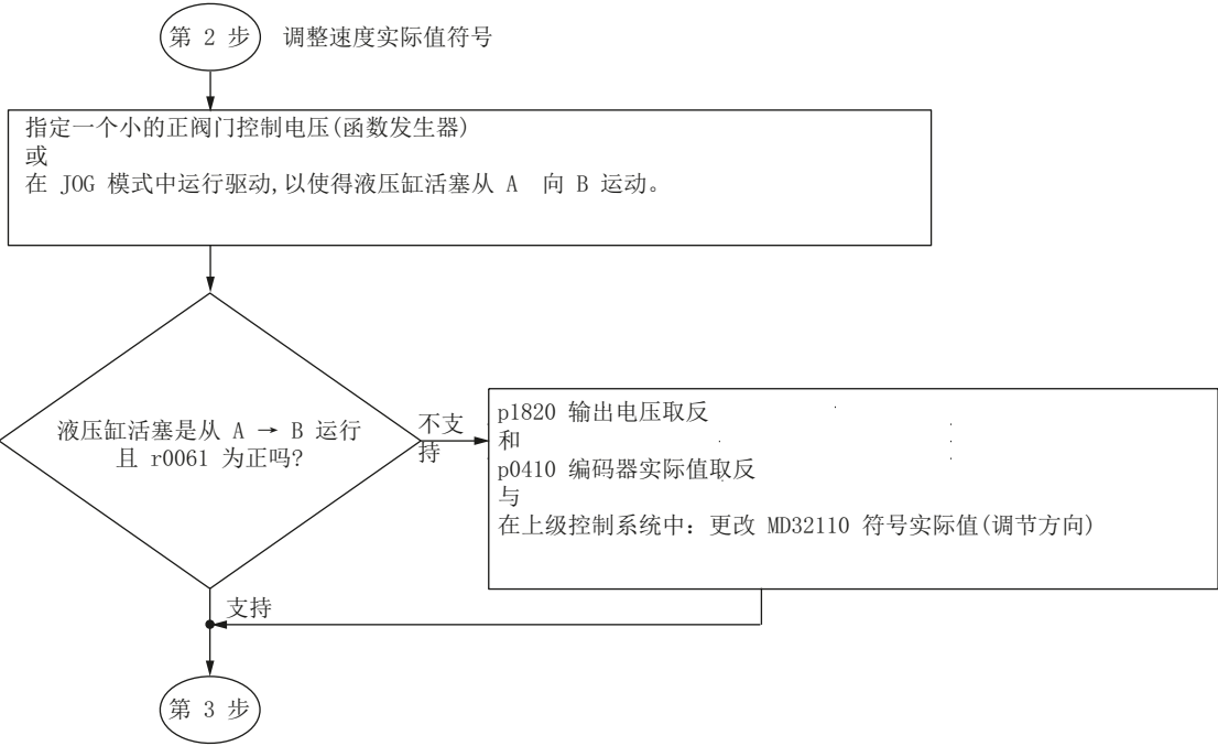
图 4-40 驱动运行方向定义的调试顺序图
