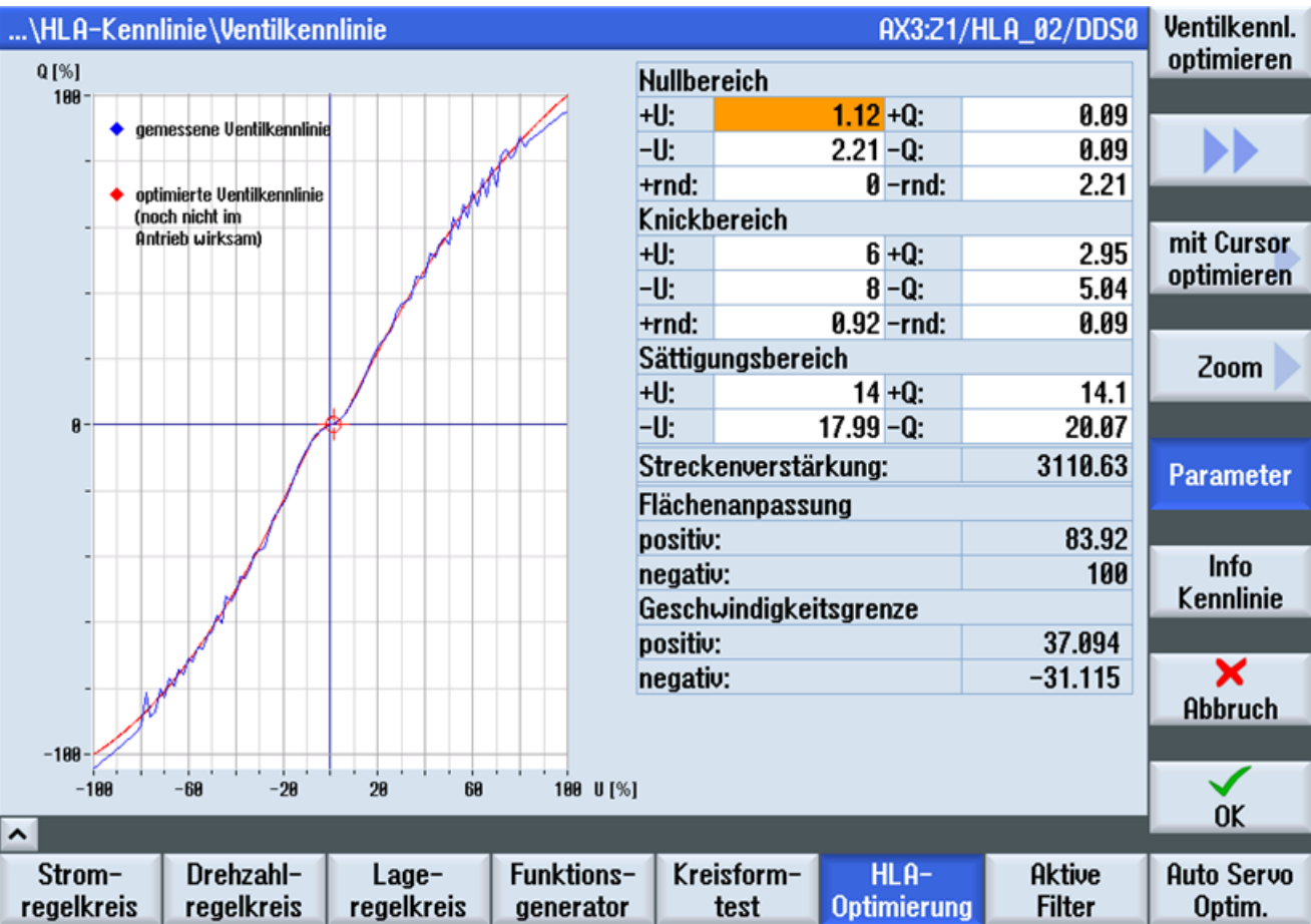
图 4-31 阀门特性曲线优化
