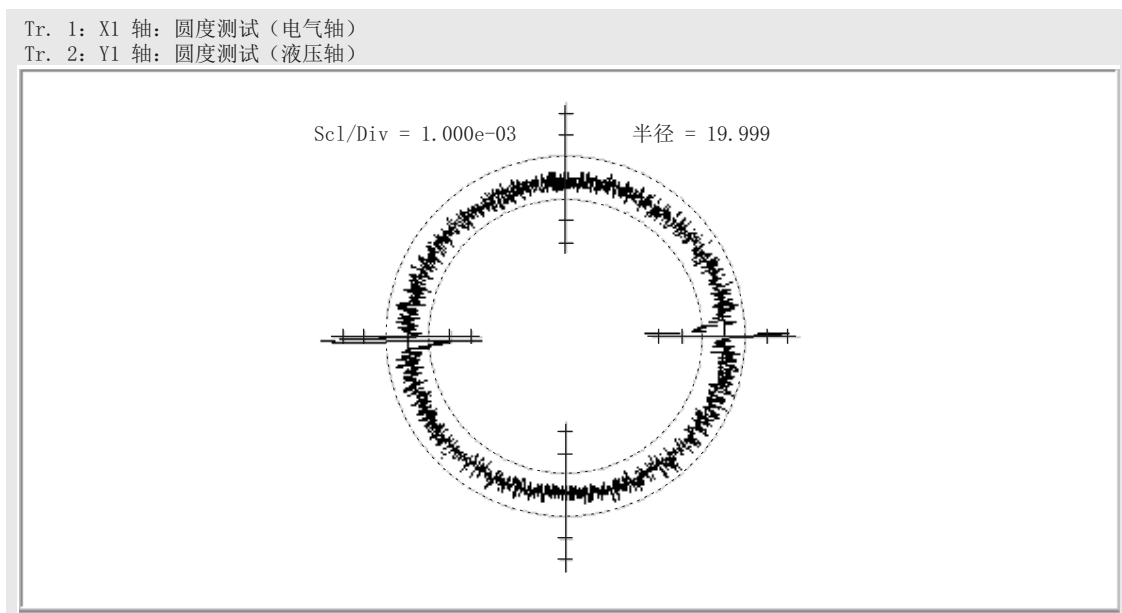
图 4-57 HRV 阀门 NG06 的圆度测试示例，15 l/min，拐点 60 %；V = 400 mm/min (运行速度)
