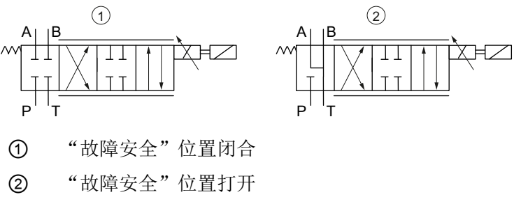
图 3-4 阀门示意图中的“故障安全”位置
