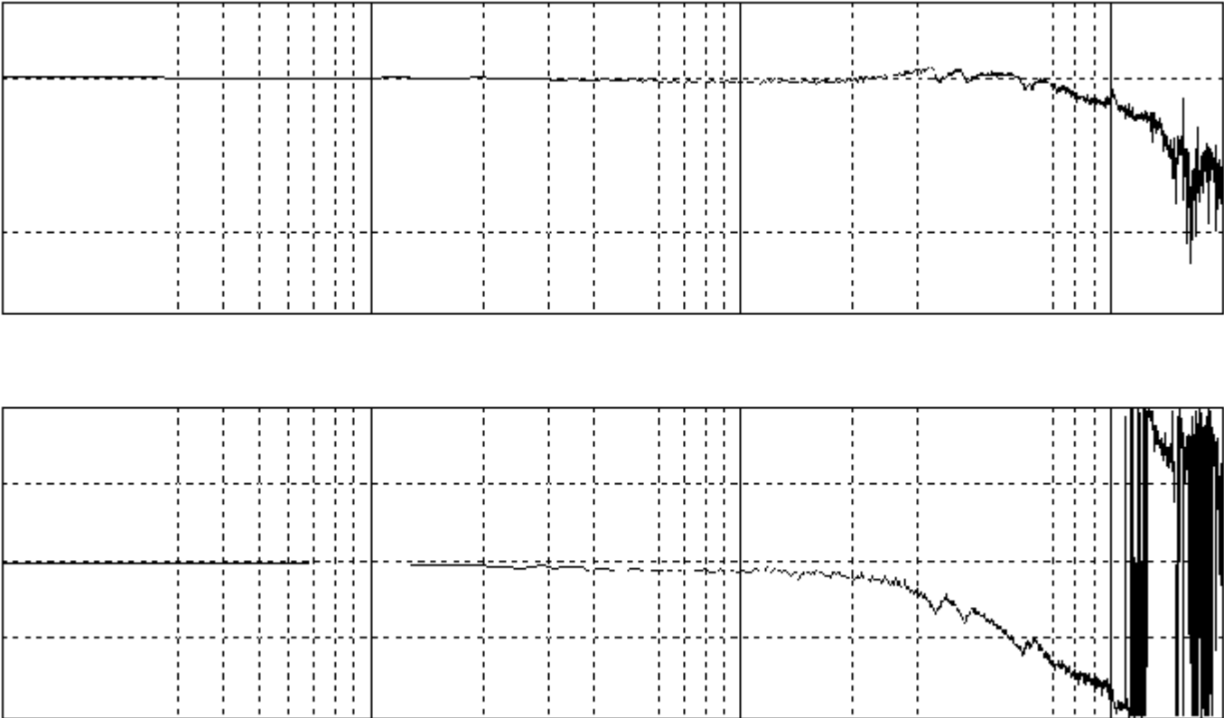
图 4-48 速度控制环参考频率响应波德图（示例）
