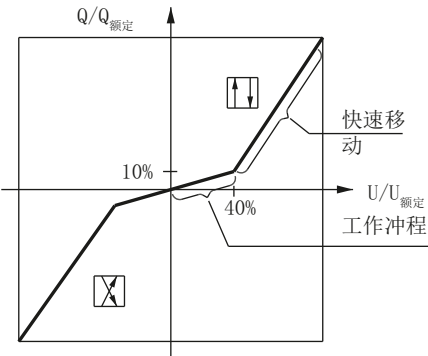
图 A-8 带拐点的体积流量特性曲线，以 40 % 的拐点为例
