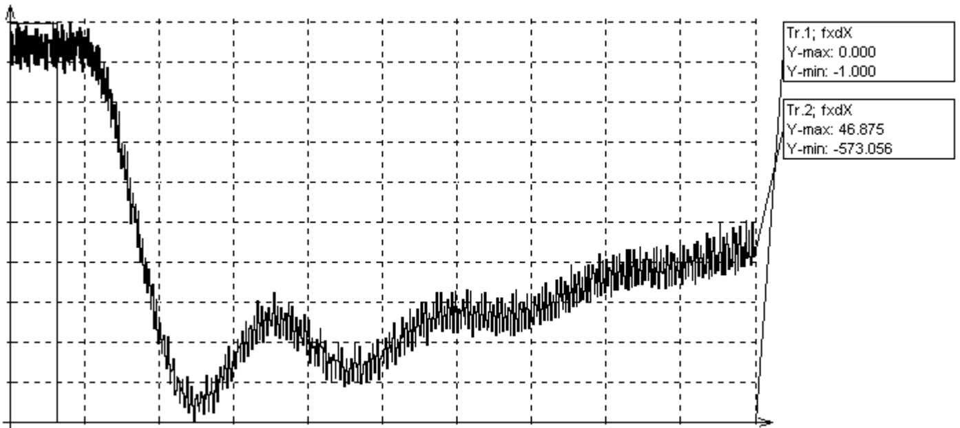
图 4-50 故障值阶跃时间特性，速度控制器积分支路（示例）
