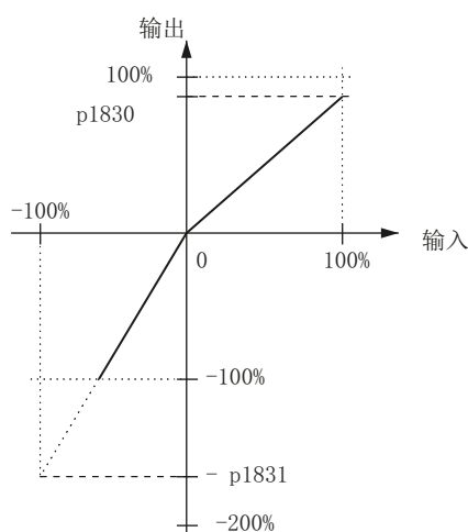
图 5-15 示例特性曲线表面补偿
