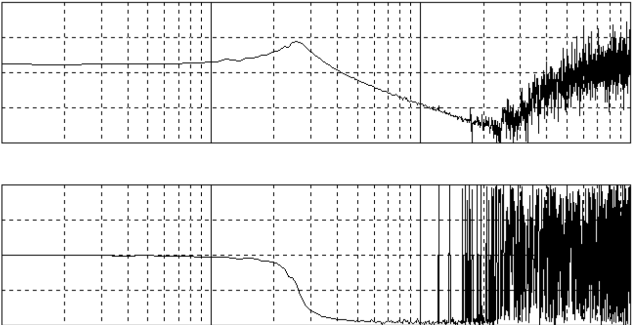
图 4-51 速度被控对象波形图 v_{\text{实际}}/Q_{\text{实际}} （示例）
