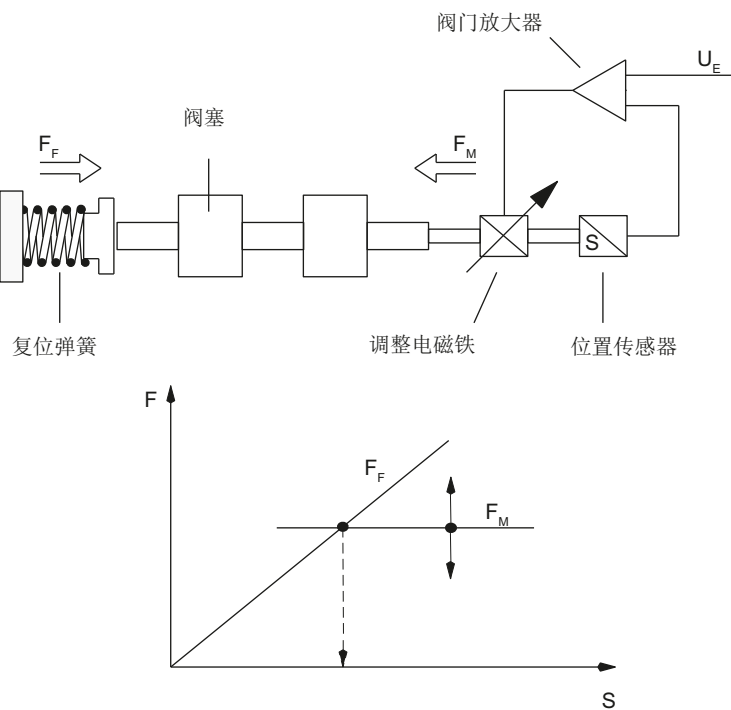
图 A-2 带阀塞位置控制的电磁控制
