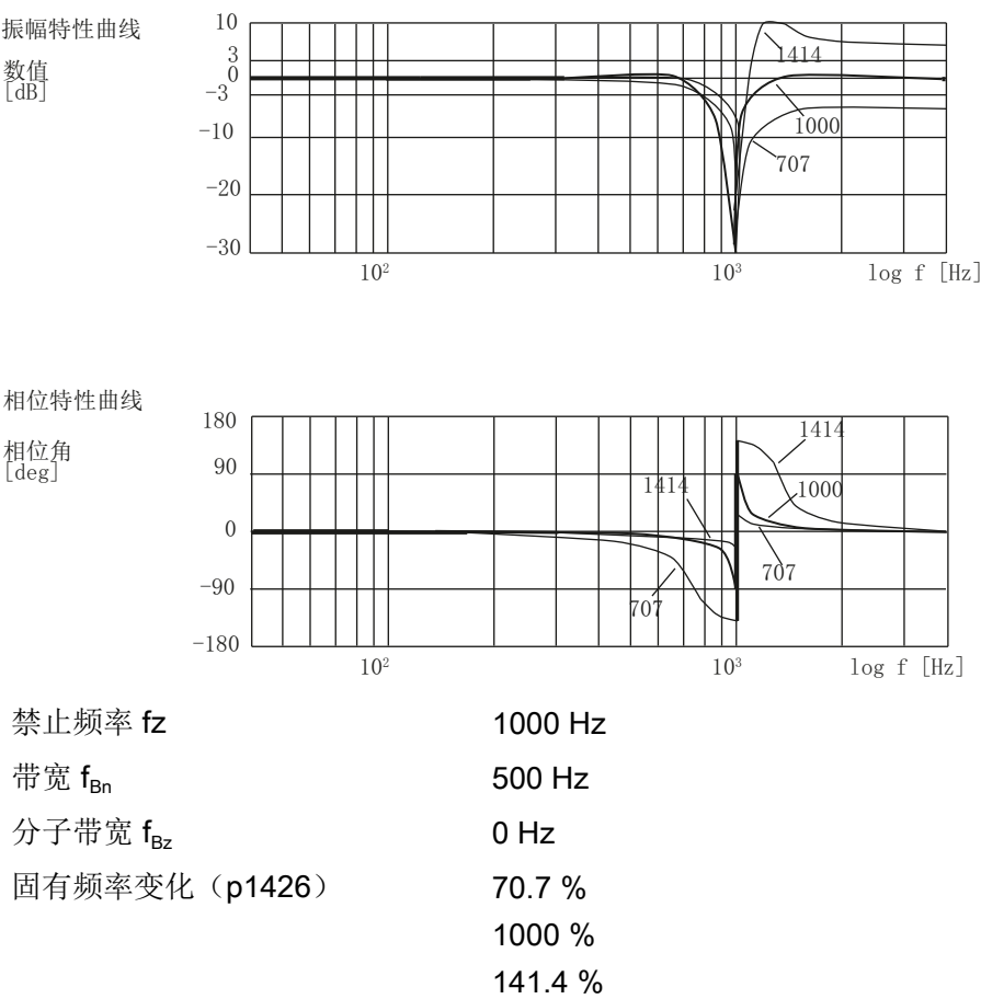
图 5-6 通用带阻的频率响应
