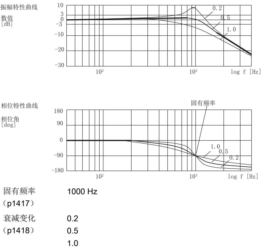
图 5-3 低通滤波器性能 (PT2)
