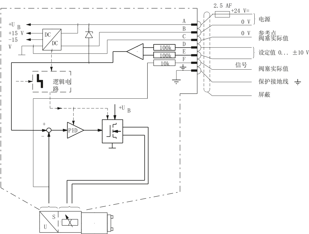
图 A-14 阀门放大器：直接控制的调节阀的方框电路图
