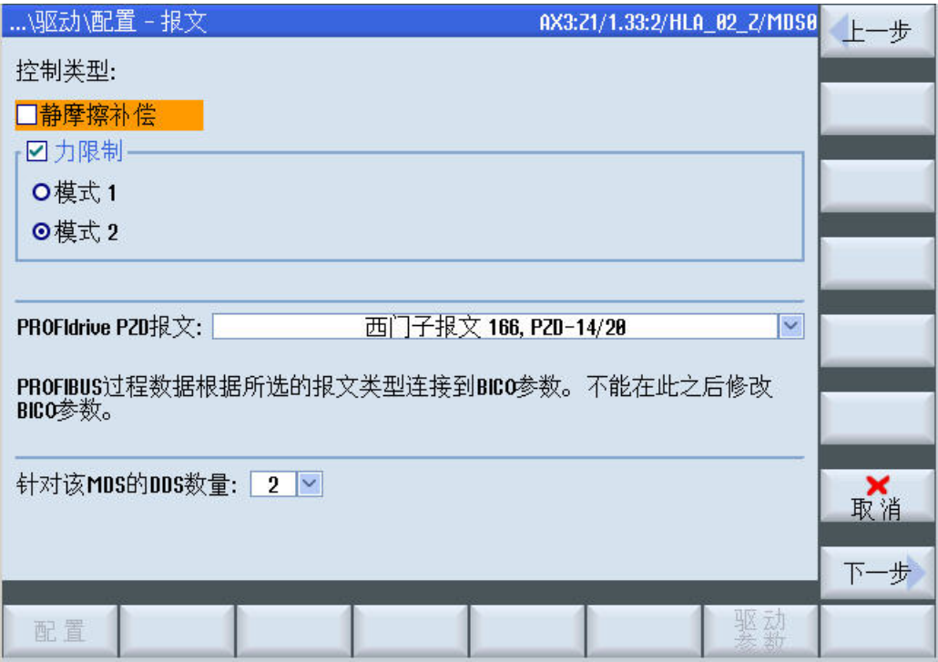
图 4-12 配置 - 控制方式/设定值
