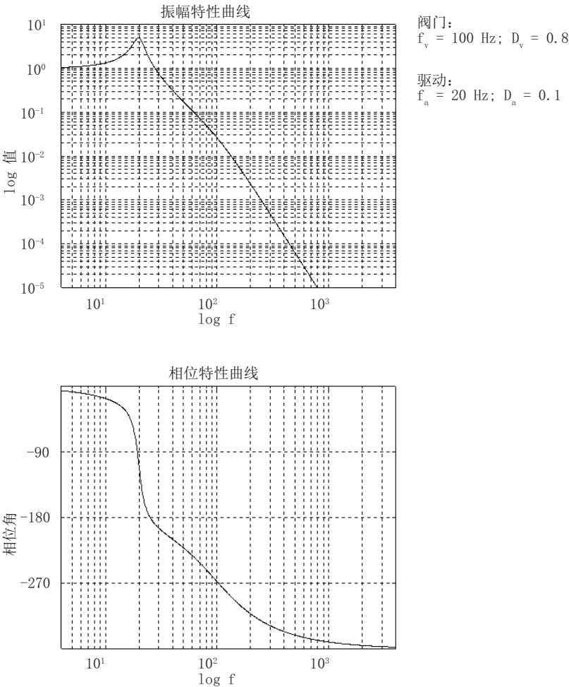
图 4-45 被控对象的频率响应特性 ( f_{\text{阀门}} \gg f_{\text{液压缸}} )
