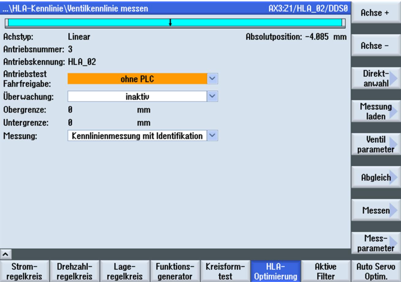
图 4-27 测量阀门特性曲线
