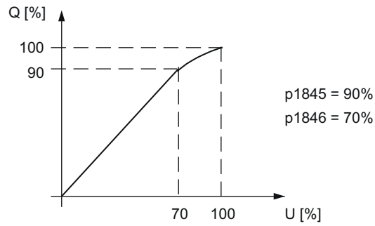
图 4-35 阀门的线性化特性曲线
