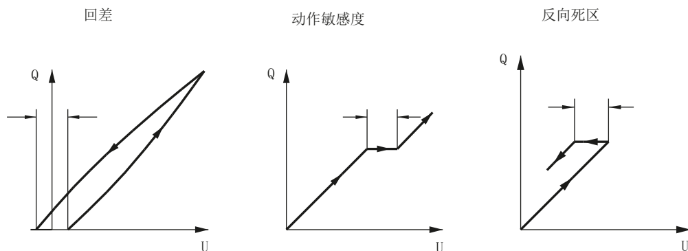
图 A-12 调节阀的回差、动作敏感度和反向死区
