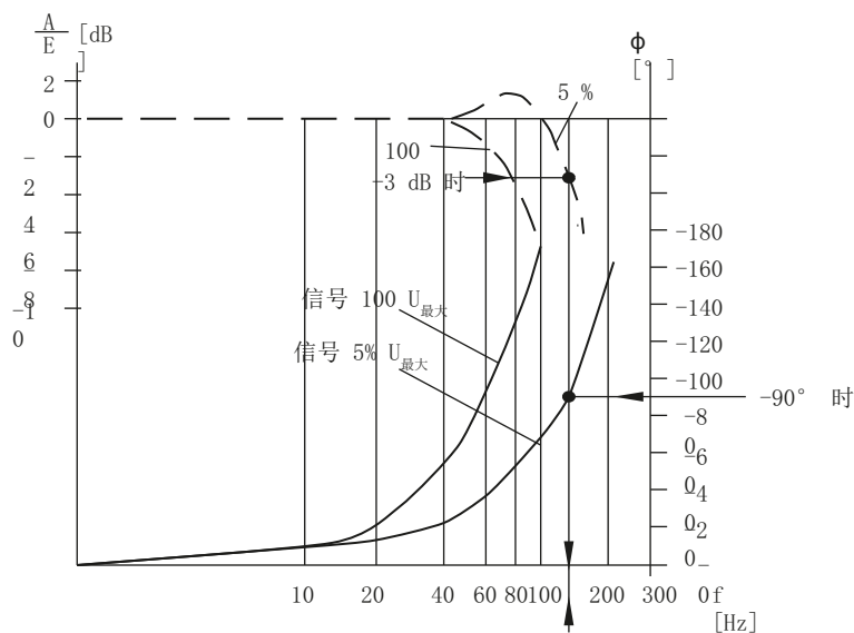
图 A-11 阀门的动态性能
