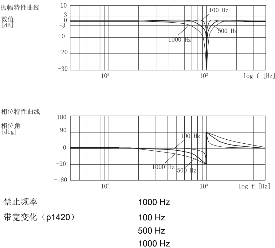
图 5-5 未衰减带阻的频率响应
