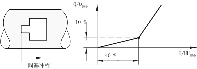
图 A-9 阀套上的阶梯状控制窗口，以 40 % 的拐点为例
