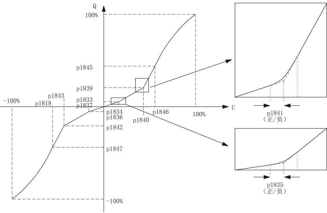
图 5-16 包含零区域、精调区域和饱和区域的折线阀门特性曲线
