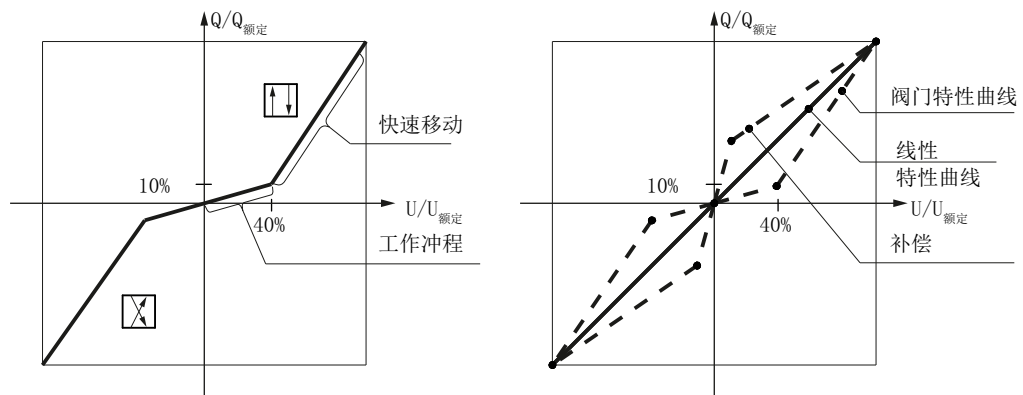
图 3-2 阀门的折线特性曲线以及 HLA 模块的补偿
