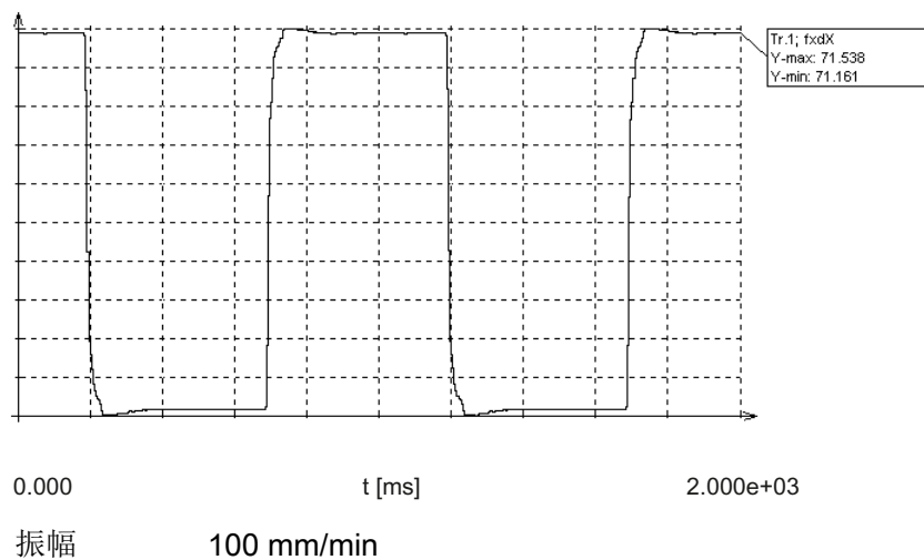
图 4-56 在信号类型为“方波”时，“位置实际值”到位置设定值的跟踪
