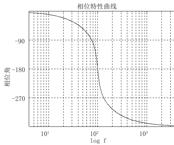
图 4-44 被控对象的频率响应特性 ( f_{\text{阀门}} \approx f_{\text{液压缸}} )
