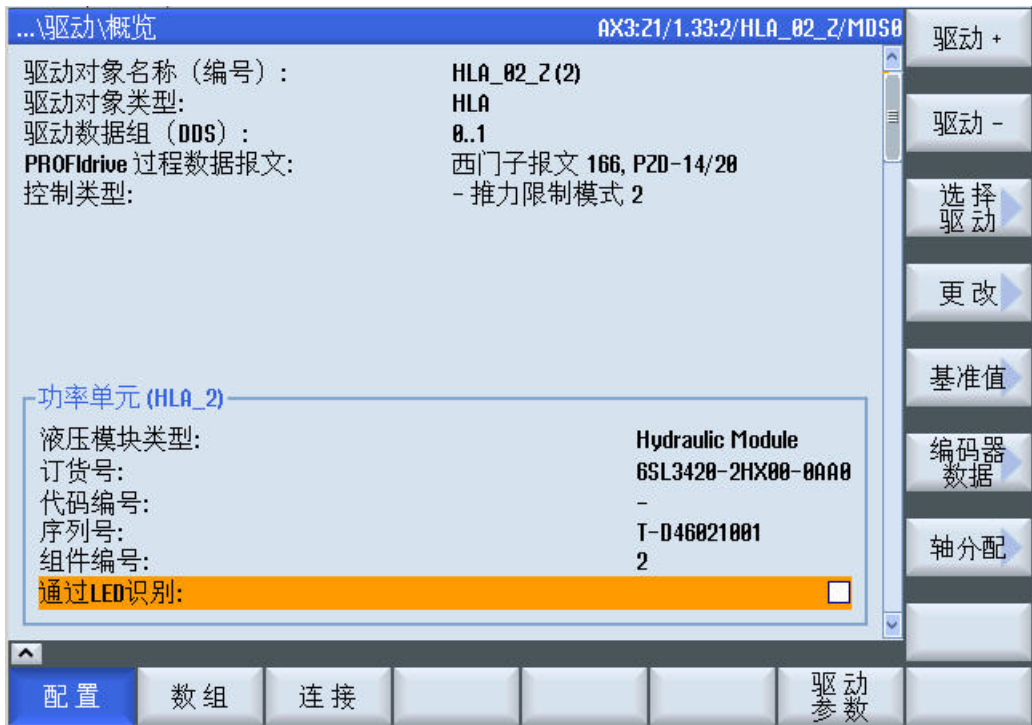
图 4-15 液压模块一览
