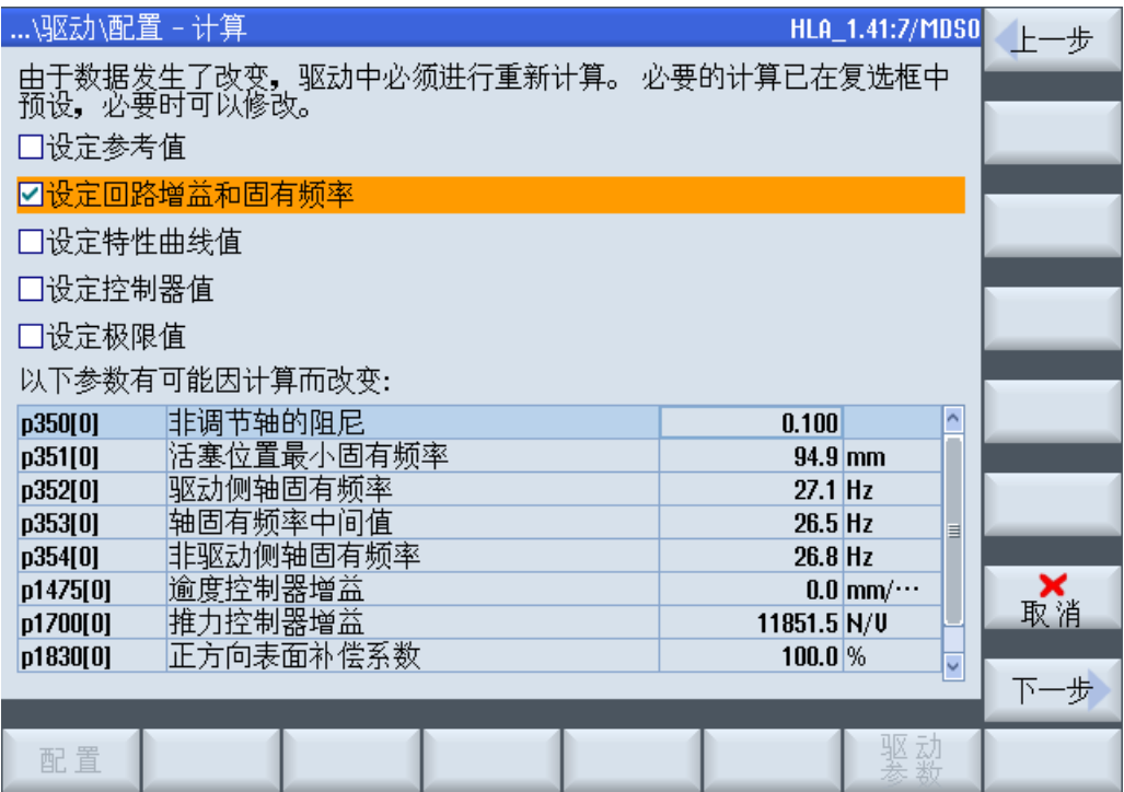
图 4-9 配置 - 计算：预设参数示例
